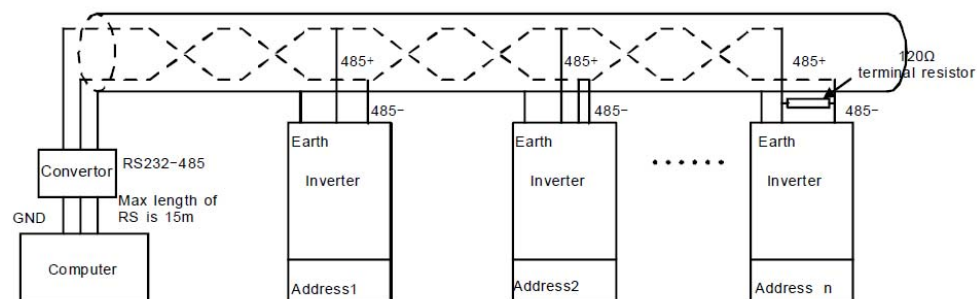
Hình 2 : Truyền nối tiếp
